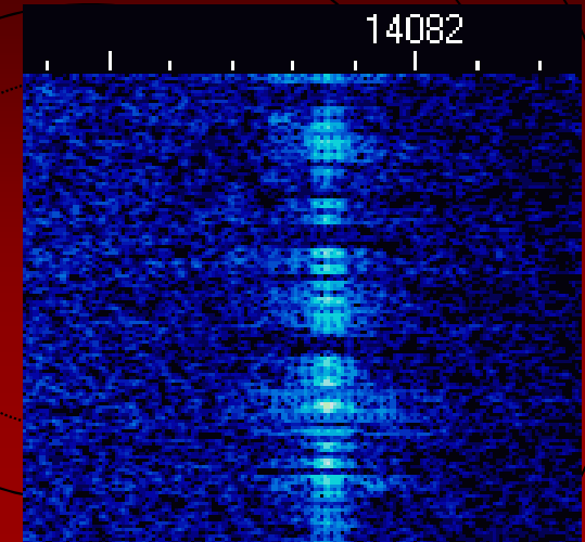
Hellschreiber Trace
