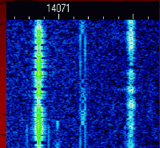
PSK31 Trace
